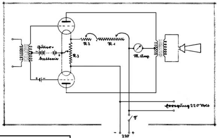
Das Schaltschema
