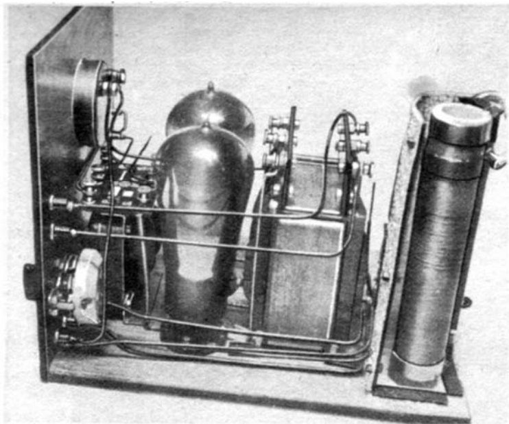
Das fertige Gerät von der Schalt- seite aus.
