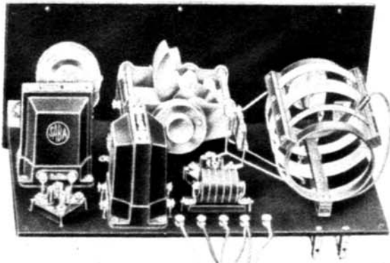
Saba-Kurzwellen-Empfänger mit 3 Röhren
