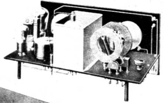
Ledion-Tropadyn 4 Röhren von Firma Vogel
