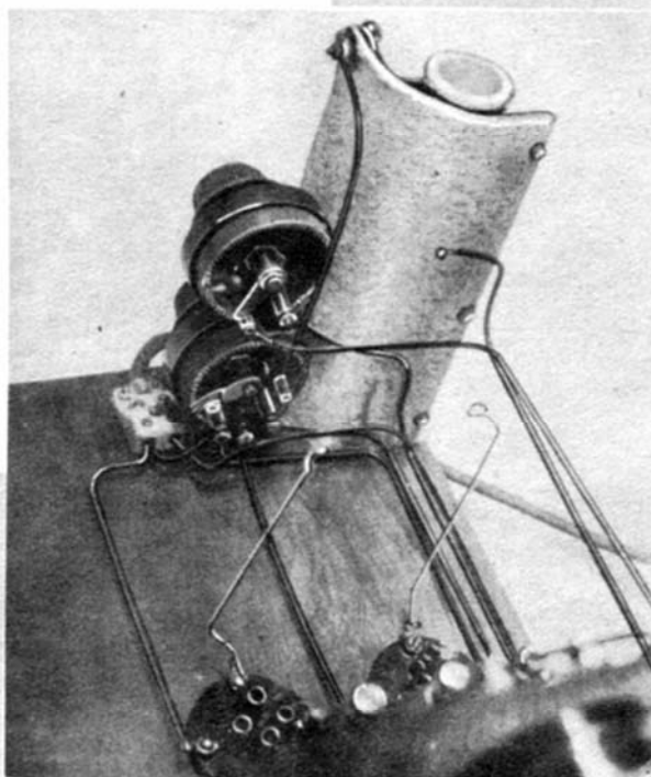
Die Leitungen zum Regulierwiderstand und zum Potentiometer. Hinter der Asbestwand der große Vorwiderstand R_1 . Beachte die Stifte am Drehwiderstand R_2 (unten), die ein Überheizen und in vollständiges Ausschalten beim Einregulieren verhindern.
