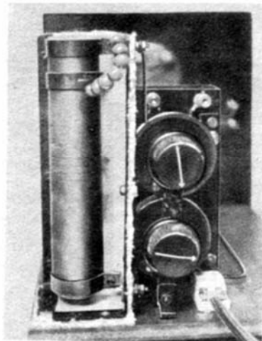
Die Widerstände und das Potentiometer
