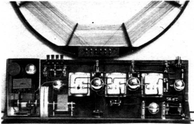
Schaleco-Schirmgittersuper mit 6 Röhren
